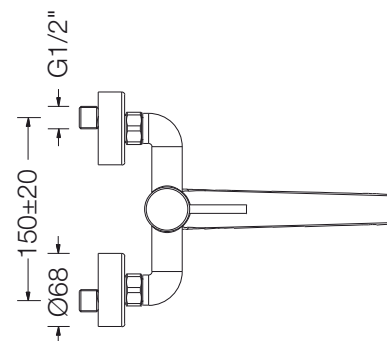
DISEGNO - DRAWING
